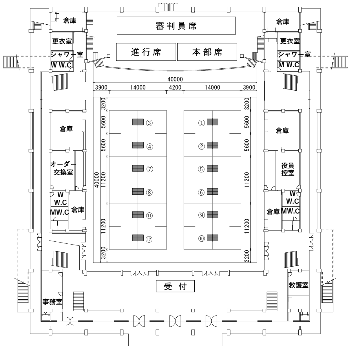
依田翁記念体育館レイアウト図 1F
