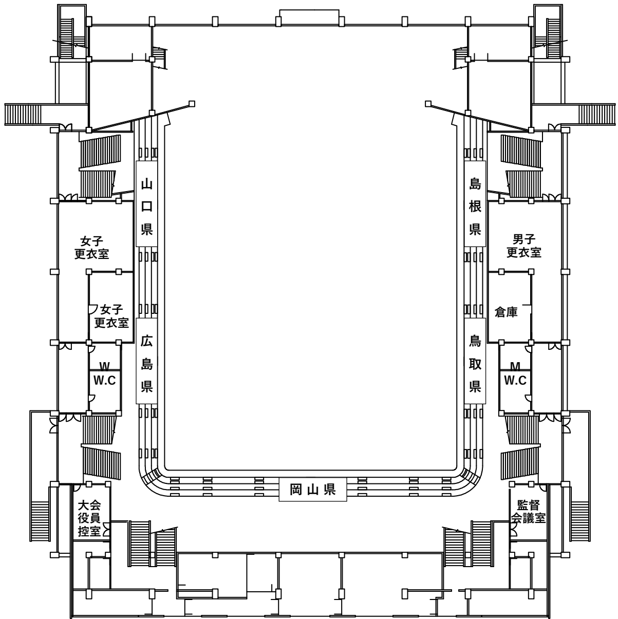
俵田翁記念体育館レイアウト図 2F
